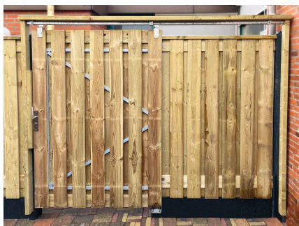
4. Ophangbeugel
